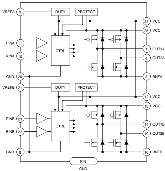
Fig. 33 BD6215FP, BD6216FP
