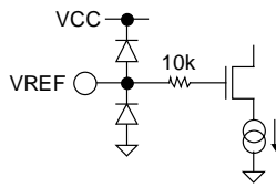
Fig.49 VREF
